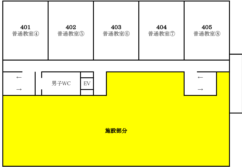
4階平面図
