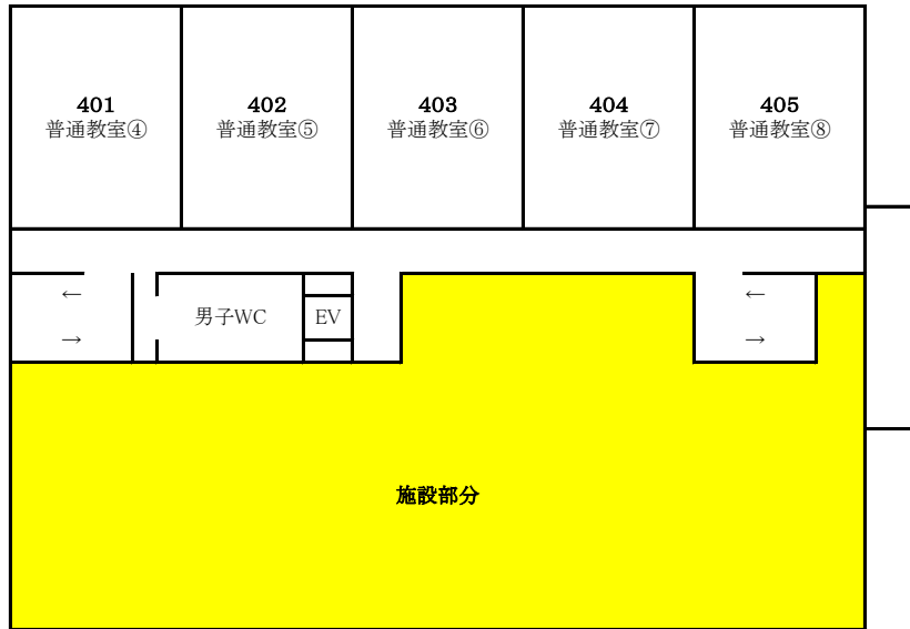
4階平面図
